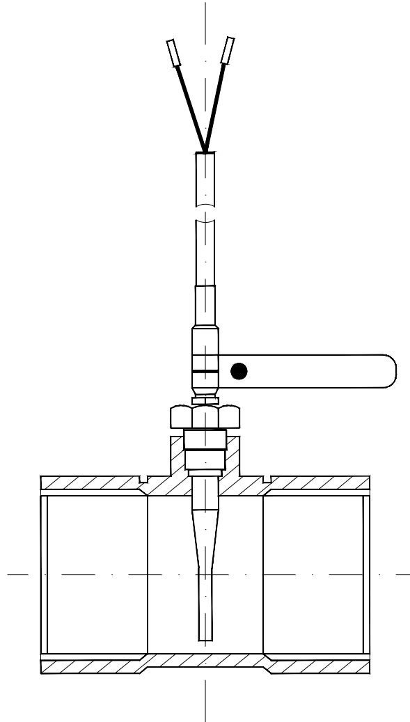
Einbau Temperaturfühler direkt eintauchend
